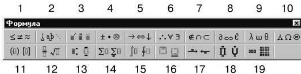
Рис. 3.1. Панель EquationEditor
